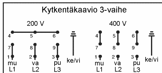
KytKentäkaavio
